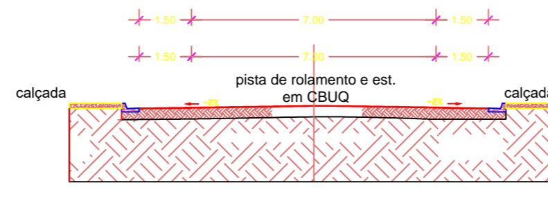
DETALHE DA SEÇÃO escala 1/150
