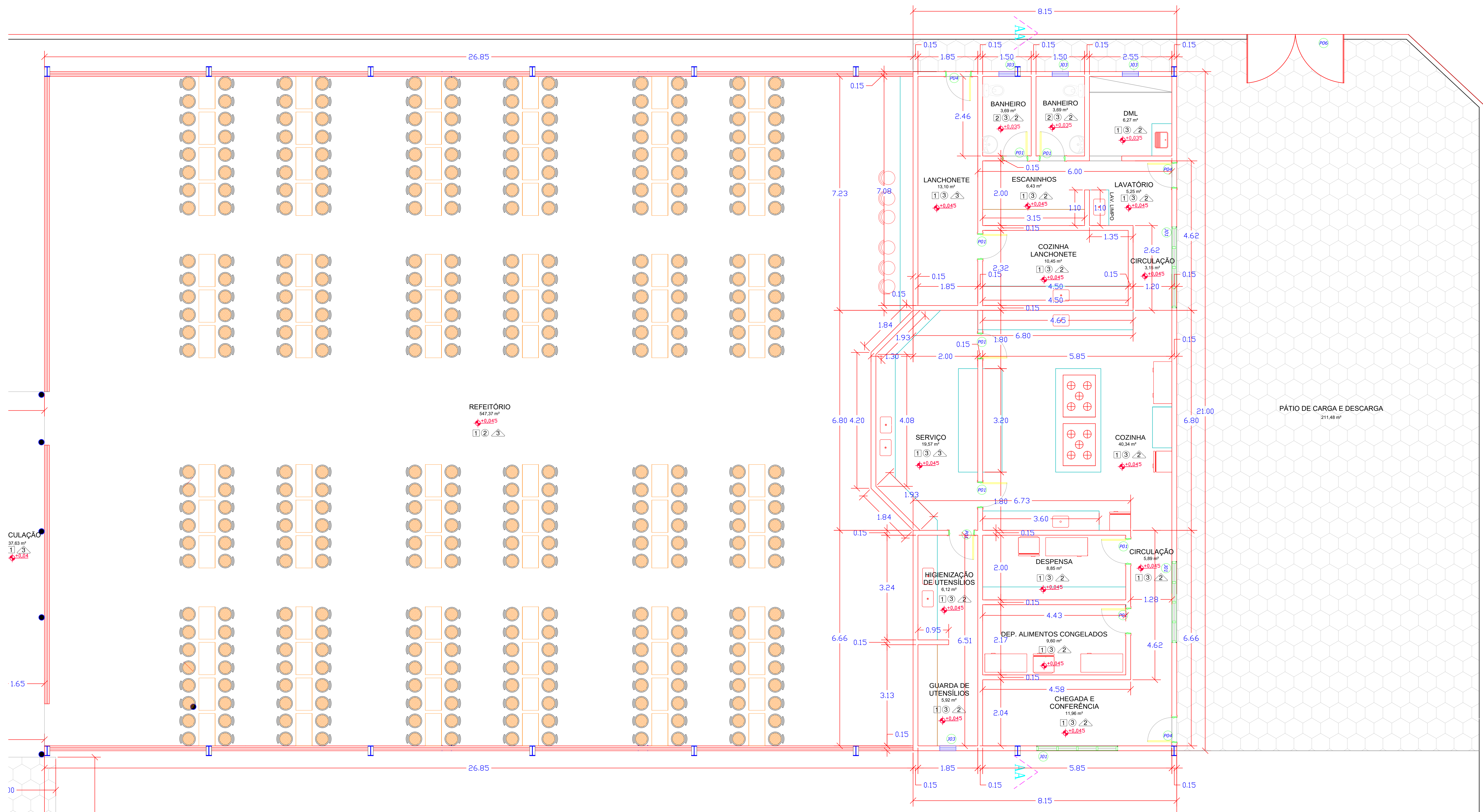
PLANTA BAIXA - REFORMA E ADAPTAÇÃO BLOCO 03
